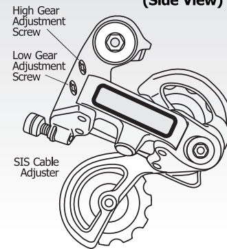
Rear Derailleur Diagram (Side View)
